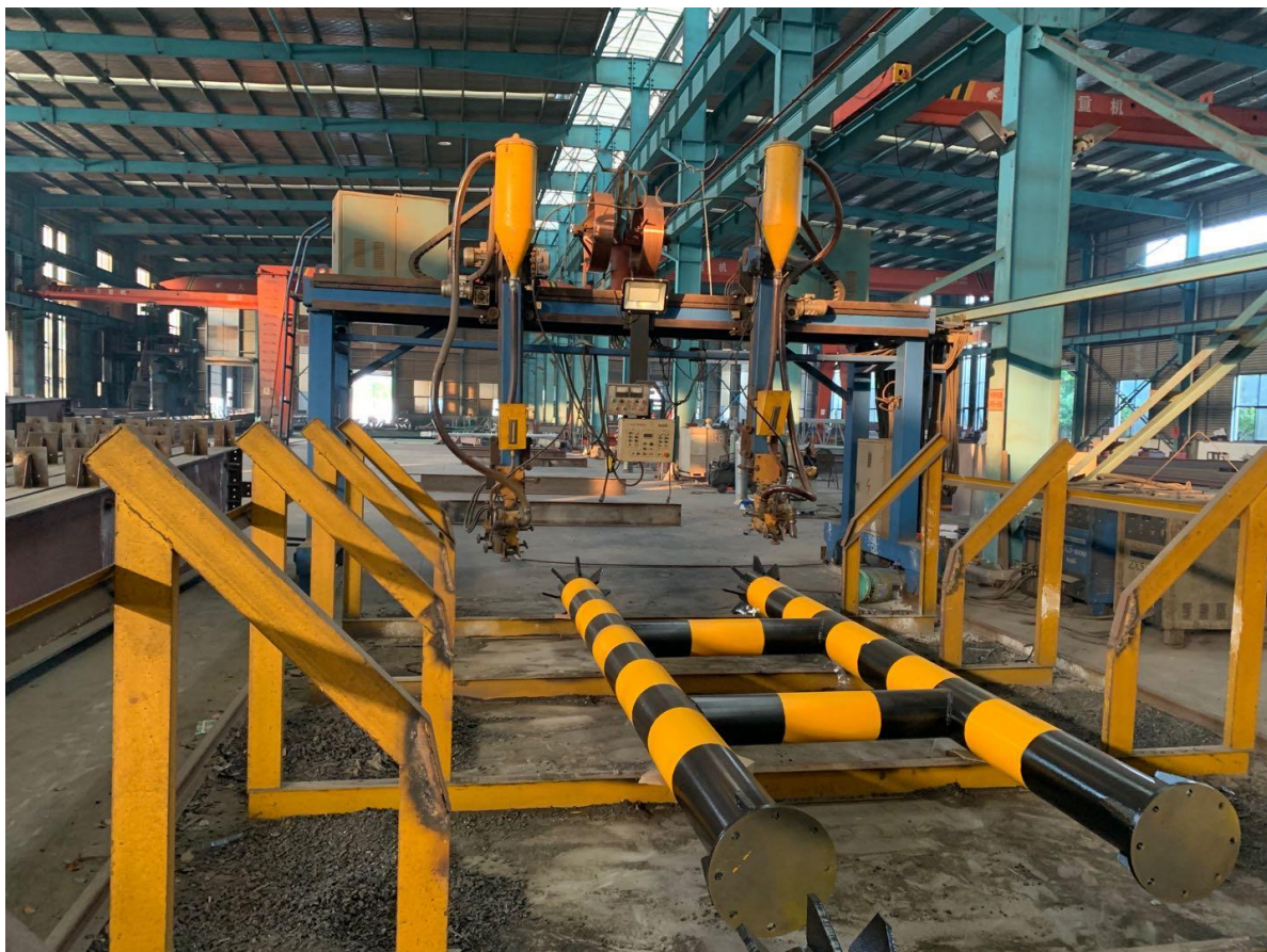
箱型自动焊接设备
